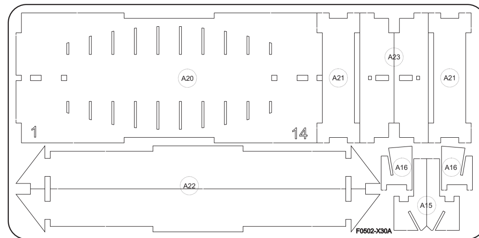
Пластина А / Plate A
