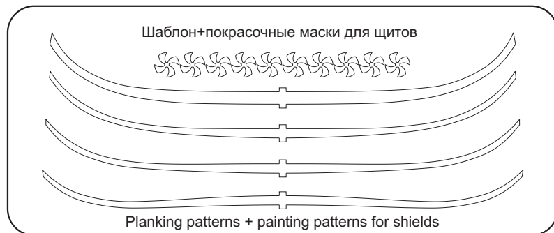
Деталь Z44 / Pattern Z44
