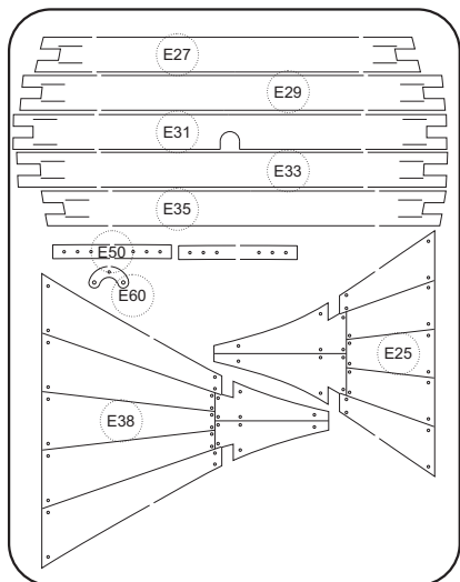
Пластина Р / Plate P
