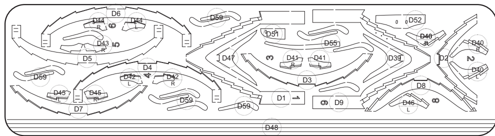
Пластина Е / Plate E
